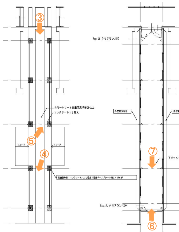
1階平面図
