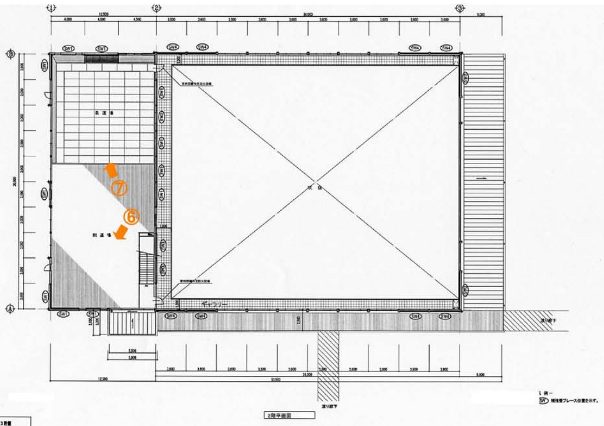
邑楽町立邑楽中学校屋内運動場耐震補強工事 補強後 2階平面図
