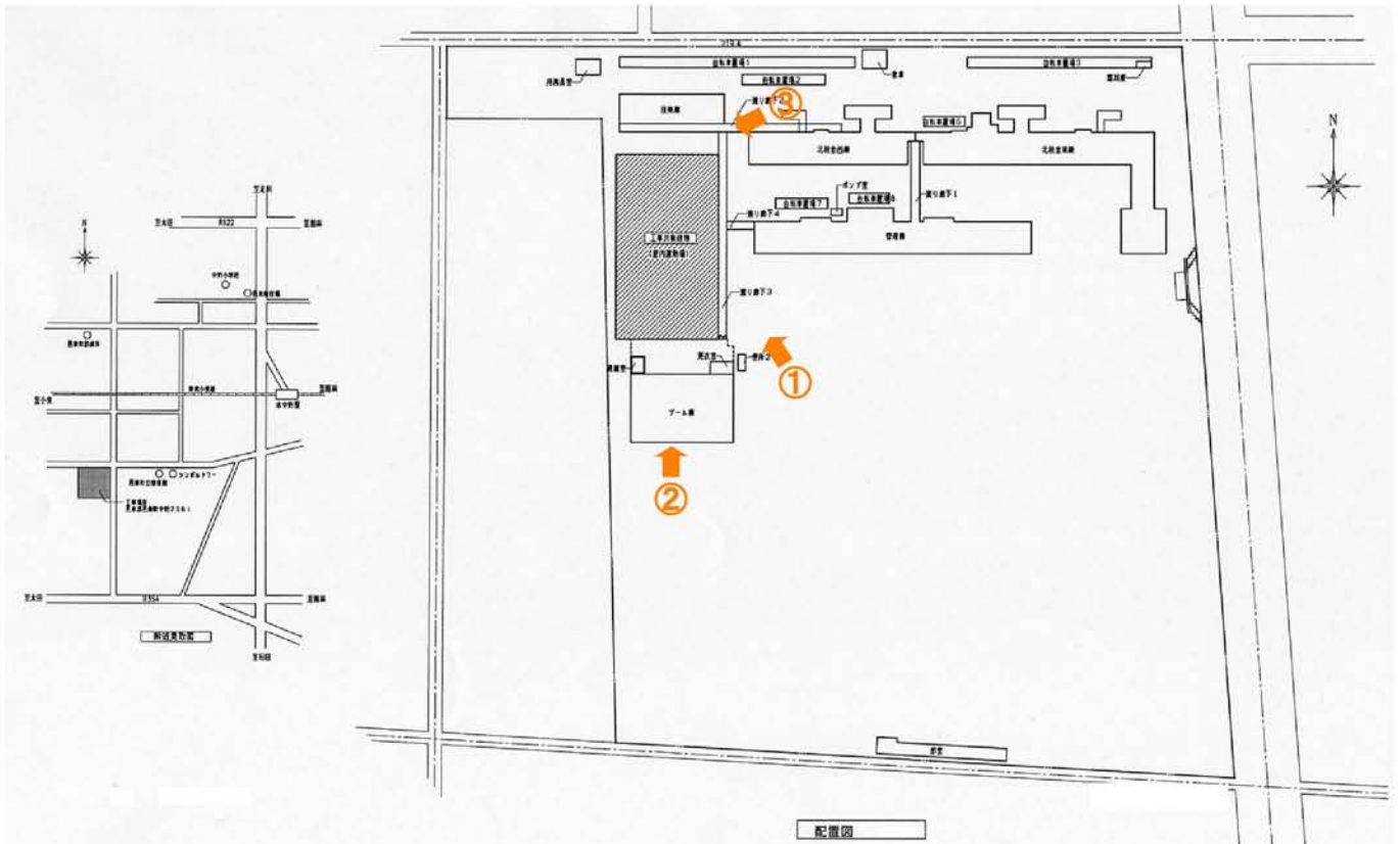
邑楽町立邑楽中学校屋内運動場耐震補強工事 配置図・附近見取図
