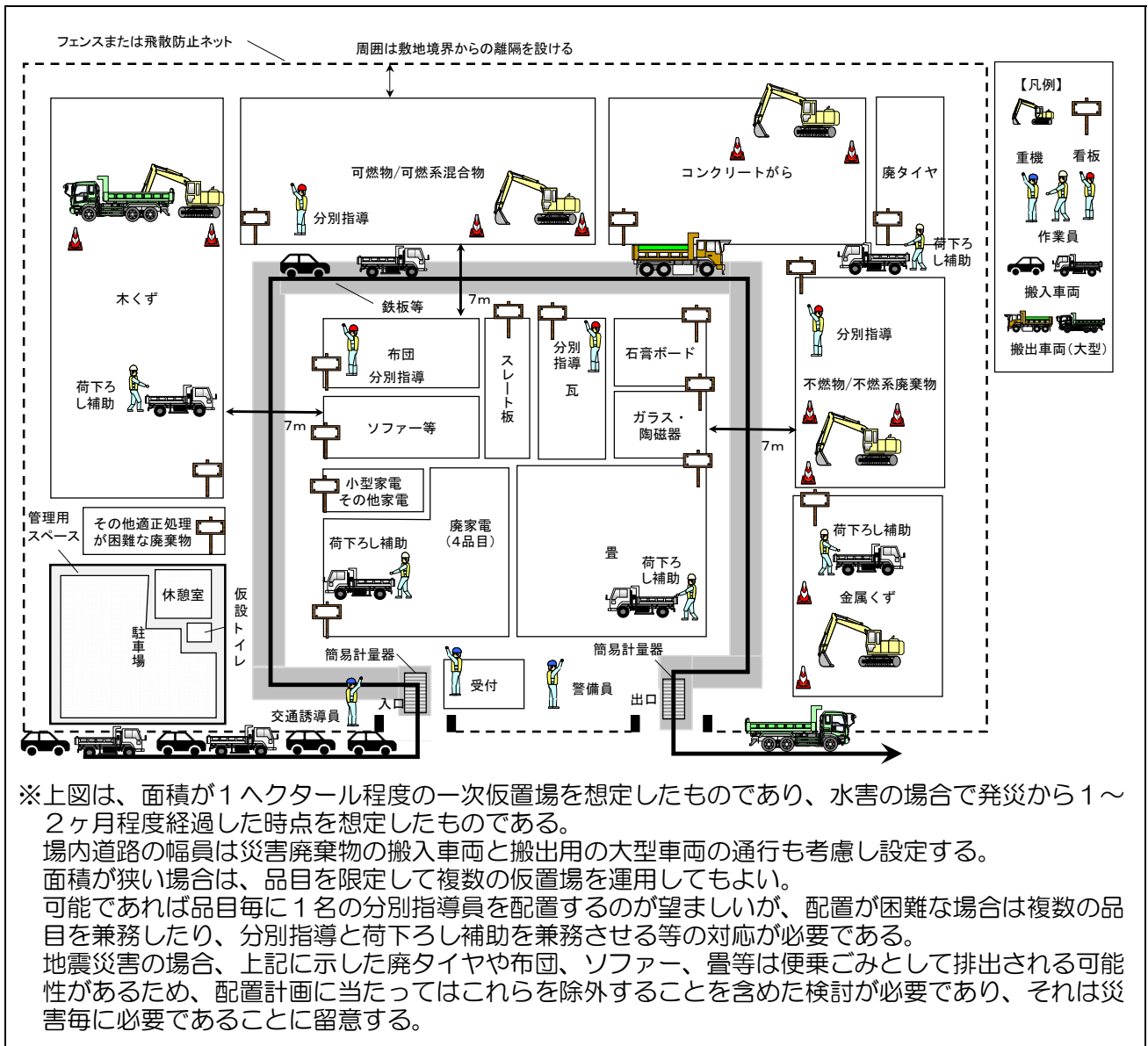
図表6-5 一次仮置場の配置計画（レイアウト）例
